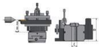
Vista posteriore Portautensili tipo H per utensili tondi
