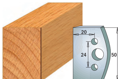
Coppia di coltelli 690.500 Coppia di limitatori 691.500
