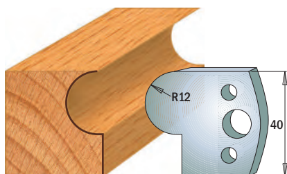
Coppia di coltelli 690.058 Coppia di limitatori 691.058
