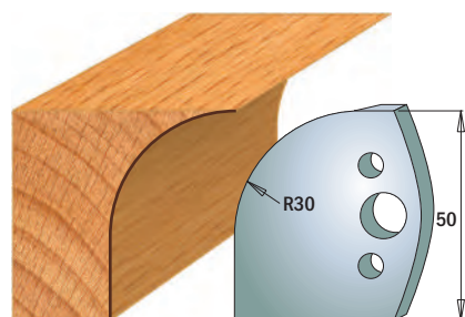
Coppia di coltelli 690.563 Coppia di limitatori 691.563
