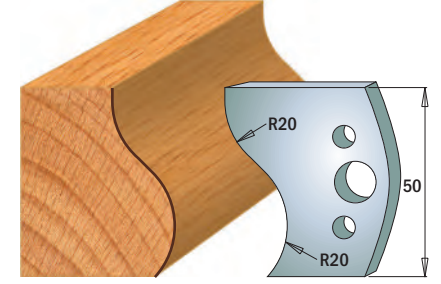
Coppia di coltelli 690.571 Coppia di limitatori 691.571
