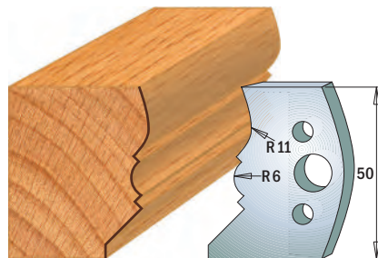
Coppia di coltelli 690.503 Coppia di limitatori 691.503
