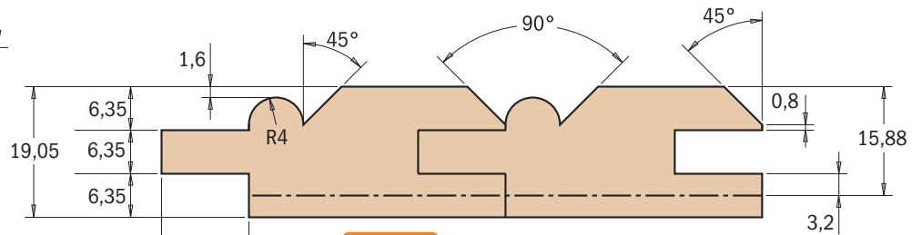
Standard con cuscinetto Ø12,7mm (791.003.00)
