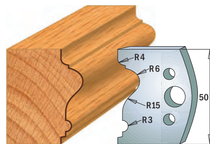
Coppia di coltelli 690.512 Coppia di limitatori 691.512
