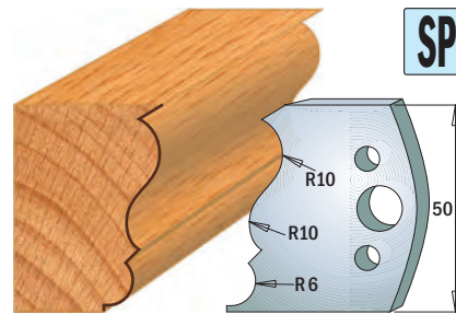
Coppia di coltelli 690.506 Coppia di limitatori 691.506
