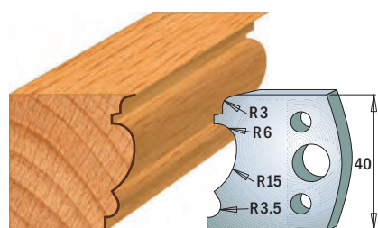
Coppia di coltelli 690.104 Coppia di limitatori 691.104
