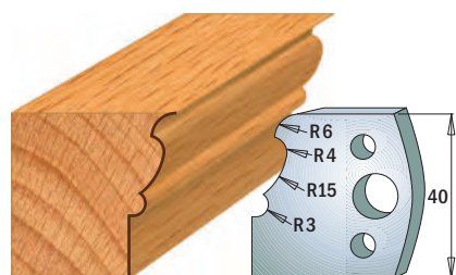
Coppia di coltelli 690.101 Coppia di limitatori 691.101
