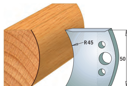
Coppia di coltelli 690.556 Coppia di limitatori 691.556
