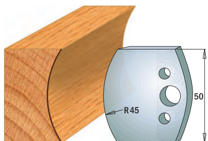
Coppia di coltelli 690.554 Coppia di limitatori 691.554
