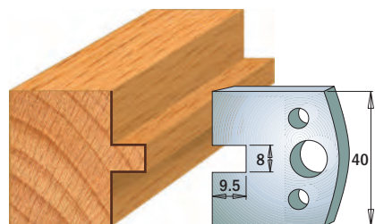
Coppia di coltelli 690.095 Coppia di limitatori 691.095
