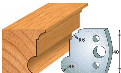
Coppia di coltelli 690.054 Coppia di limitatori 691.054
