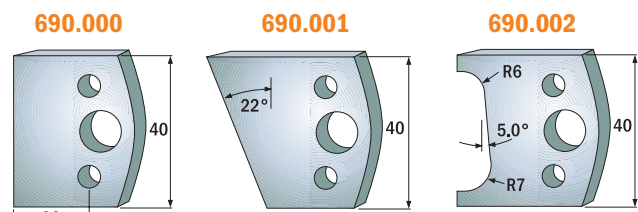
Coltelli sagomati, lunghezza di taglio=40mm (serie 690)
