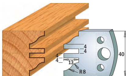
Coppia di coltelli 690.097 Coppia di limitatori 691.097
