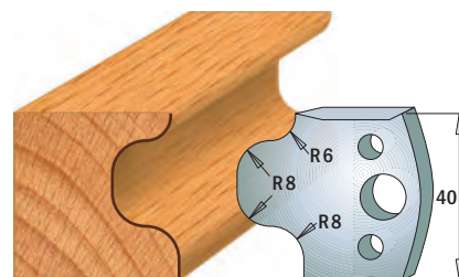
Coppia di coltelli 690.056 Coppia di limitatori 691.056
