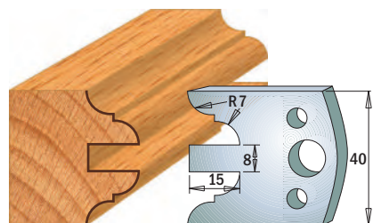
Coppia di coltelli 690.098 Coppia di limitatori 691.098
