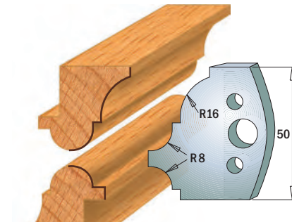
Coppia di coltelli 690.541 Coppia di limitatori 691.541
