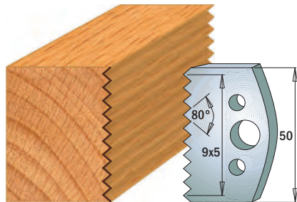
Coppia di coltelli 690.524 Coppia di limitatori 691.524
