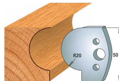
Coppia di coltelli 690.562 Coppia di limitatori 691.562
