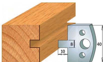
Coppia di coltelli 690.094 Coppia di limitatori 691.094
