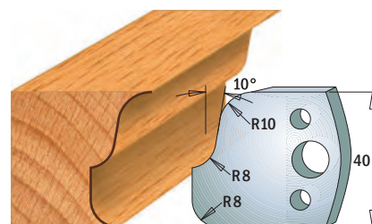
Coppia di coltelli 690.059 Coppia di limitatori 691.059
