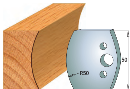
Coppia di coltelli 690.560 Coppia di limitatori 691.560
