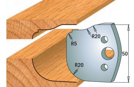
Coppia di coltelli 690.577 Coppia di limitatori 691.577
