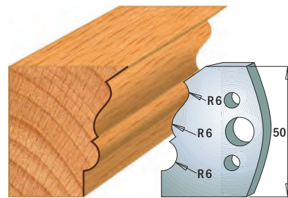
Coppia di coltelli 690.509 Coppia di limitatori 691.509
