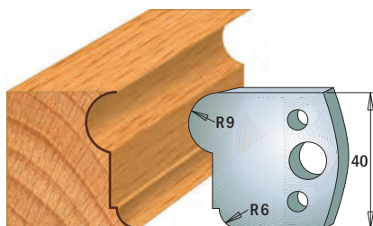
Coppia di coltelli 690.055 Coppia di limitatori 691.055
