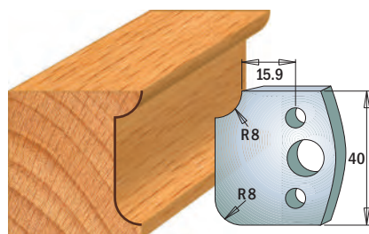
Coppia di coltelli 690.174 Coppia di limitatori 691.174
