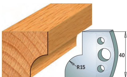
Coppia di coltelli 690.057 Coppia di limitatori 691.057
