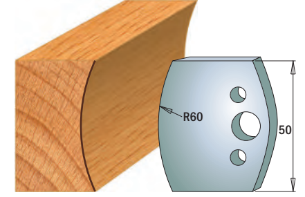
Coppia di coltelli 690.574 Coppia di limitatori 691.574
