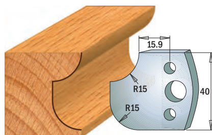
Coppia di coltelli 690.177 Coppia di limitatori 691.177
