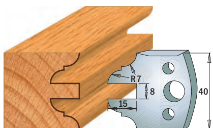
Coppia di coltelli 690.099 Coppia di limitatori 691.099
