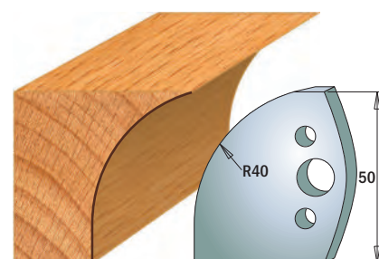
Coppia di coltelli 690.565 Coppia di limitatori 691.565
