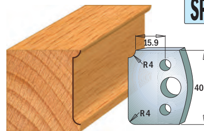
Coppia di coltelli 690.171 Coppia di limitatori 691.171
