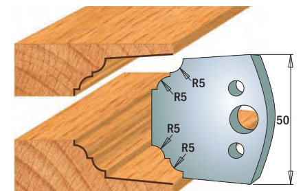
Coppia di coltelli 690.580 Coppia di limitatori 691.580
