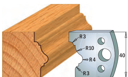
Coppia di coltelli 690.102 Coppia di limitatori 691.102
