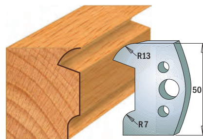
Coppia di coltelli 690.518 Coppia di limitatori 691.518
