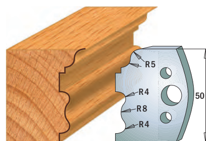
Coppia di coltelli 690.515 Coppia di limitatori 691.515
