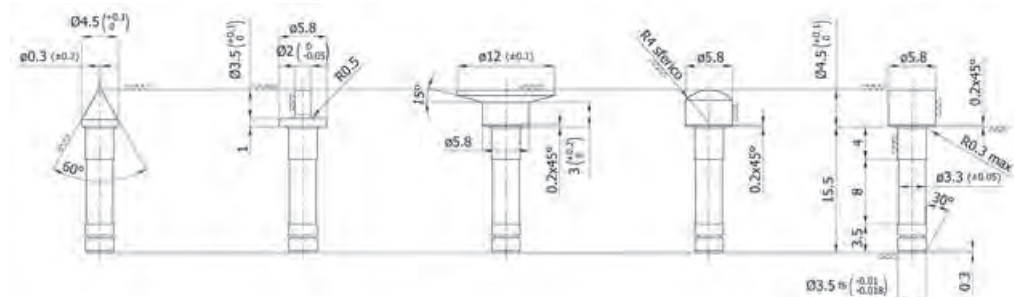
E - Insetto conico Point anvil D - Insetto cilindrico Spline anvil C - Insetto a piattello Disc anvil B - Insetto sferico Spherical anvil A - Insetto piatto Flat anvil
